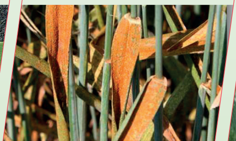
Кафява/листна ръжда
